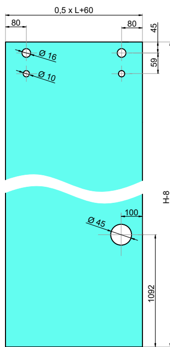
glass door
